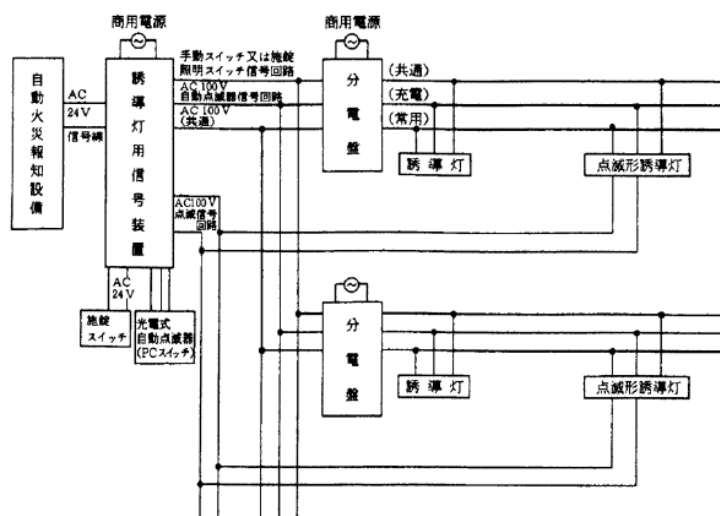
圖16-23 機器結線圖
